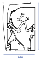
B27 ELITE / PRESTIGE montage au plafond
