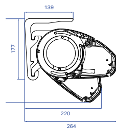
B50 XL montage au plafond
