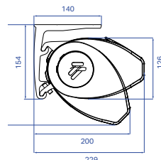
B50 S montage au plafond
