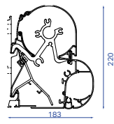
B25 ELITE / PRESTIGE VOLANT montage murale
