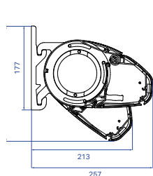
B50 XL montage murale
