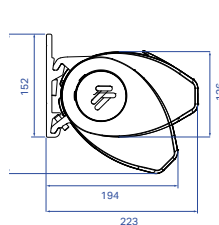
B50 S montage murale
