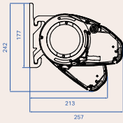
Montage mural
