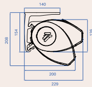
Montage plafond
