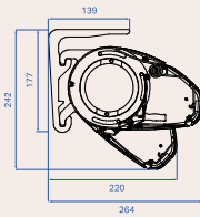
Montage plafond
