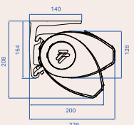
Montage plafond
