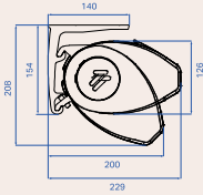
Montage plafond
