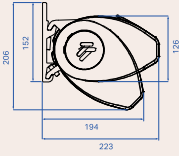
Montage mural
