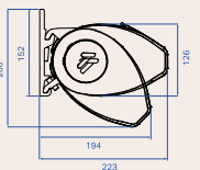
Montage mural
